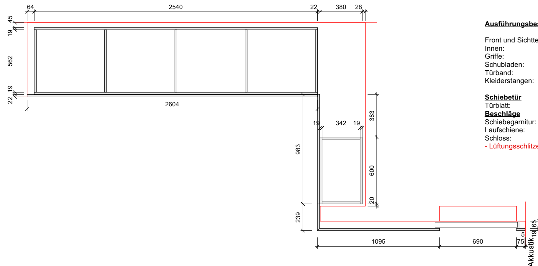
C-C Sockelplan
